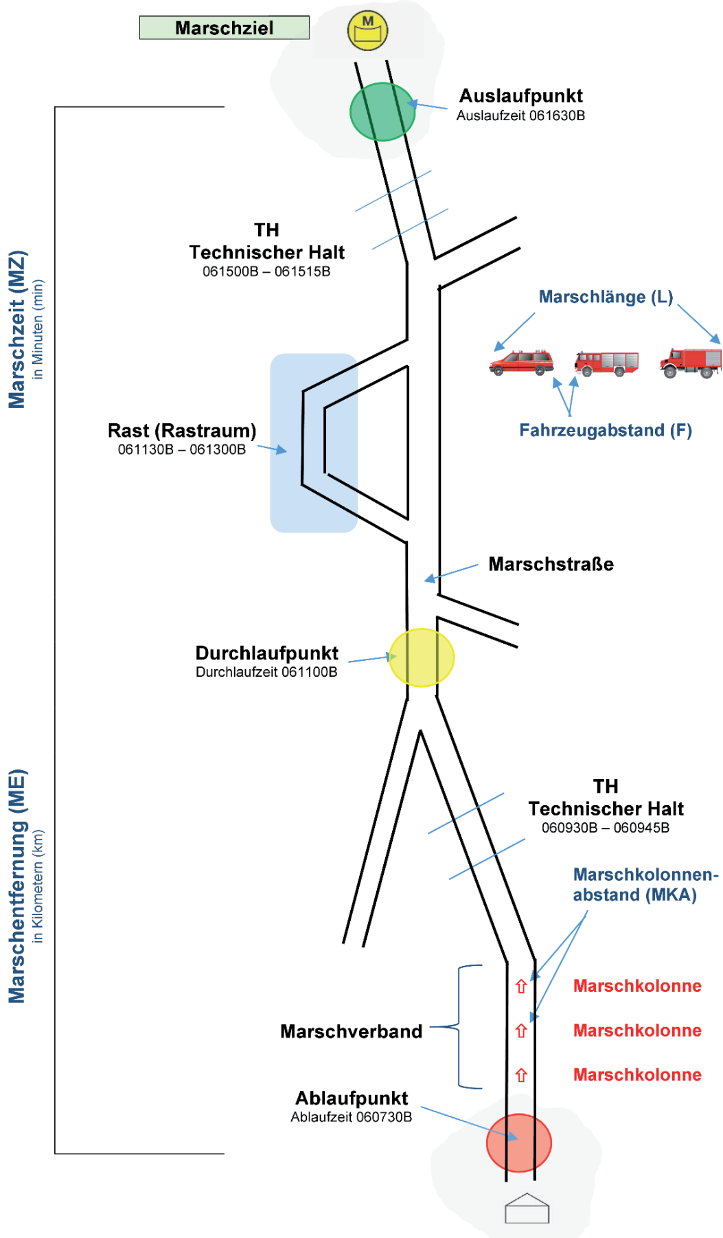
Abbildung 1 - Schematische Darstellung der Fachbegriffe
